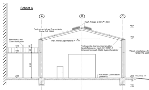
Schnitt
